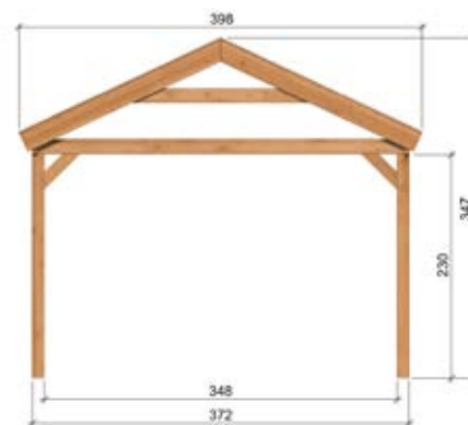
Zijaanzicht
