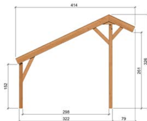
Zijaanzicht
