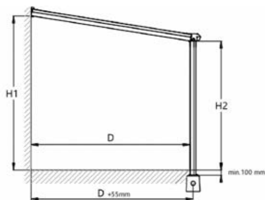
Tekening zijkant
