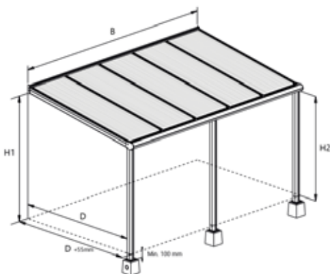
Tekening 3D
