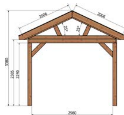
Zijaanzicht L
